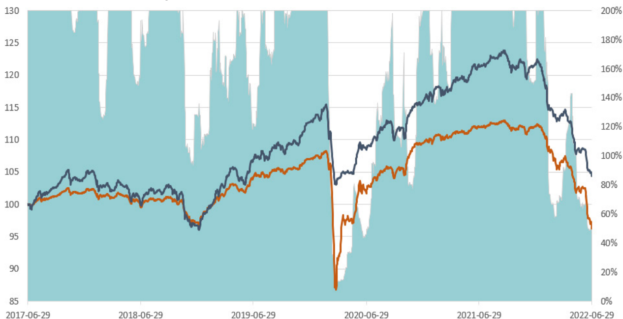
Simulerad historisk kursutveckling, normaliserad: 2017-06-29 - 2022-06-29
